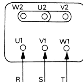
Conexión Estrella
